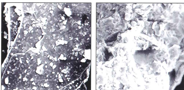
湿潤性(親水性)土壌粒子の電子顕微鏡写真。腐植物質がほとんどないことが明白である。非湿潤性(疎水性)土壌粒子の電子顕微鏡写真。腐植物質の交互積層堆積が明白である。
