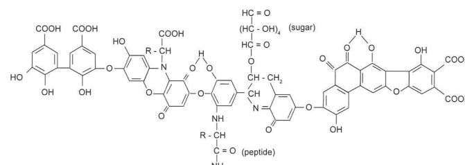
腐植酸のモデル構造図 (Stevenson 1982)
